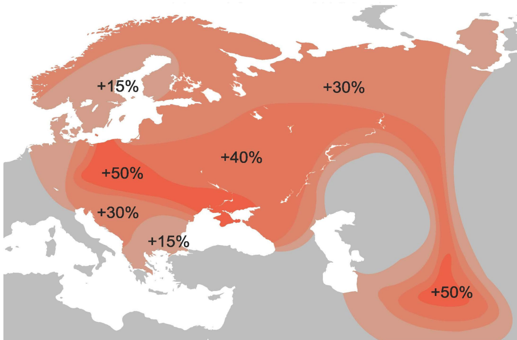
Рис. 1 - Частота распределения R1a, Википедия, статья «Гаплогруппа R1a (Y-ДНК)».
